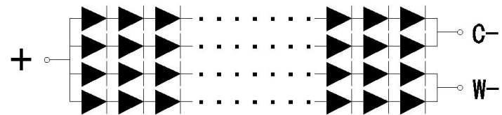
等效电路 (2 并 13 串*2) Equivalent-circuit (2 parallels 13 series*2)
