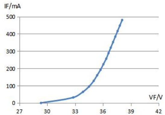
4、伏安特性曲线 Voltage Vs Current
