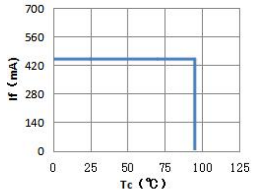
2、Tc-If 曲线图 TC VS IF curve
