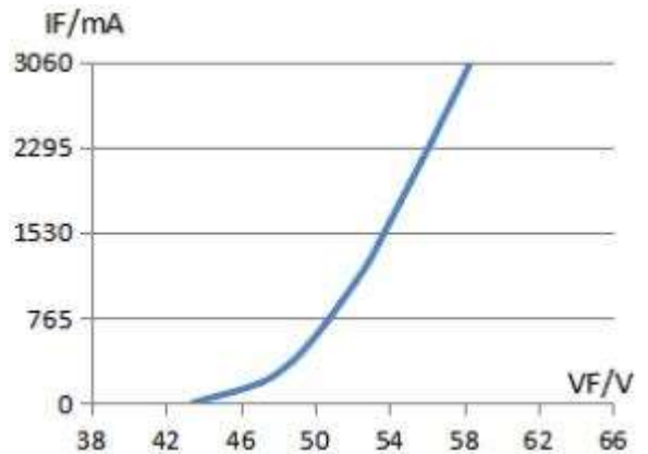
4、伏安特性曲线 Voltage Vs Current
