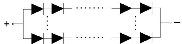
等效电路（6并12串）
