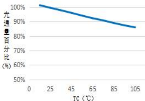
1、温度与光通量曲线图 Temperature Vs Lumen
