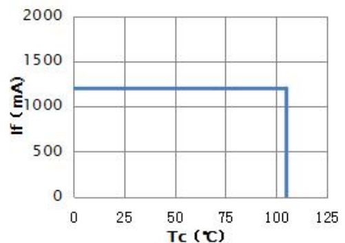
2、T c -I f 曲线图 T C VS I F curve
